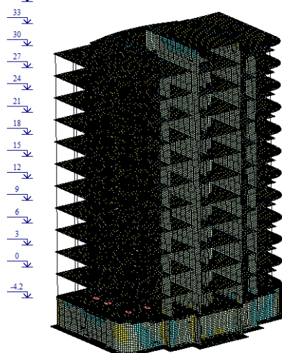
Рис. 2 Мозаика напряжений по M_x
