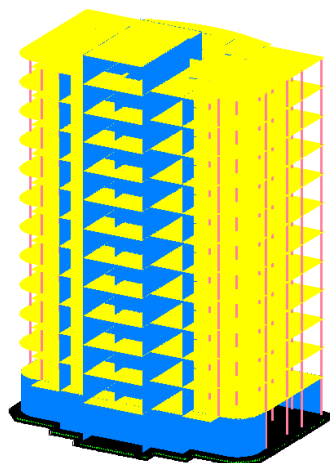
Рис. 1 Мозаика назначенных материалов ЖБ
